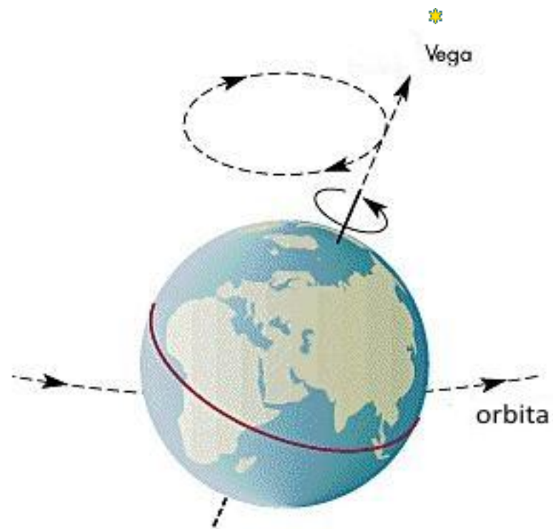
Rotacija Zemlje pred 14.000leti
