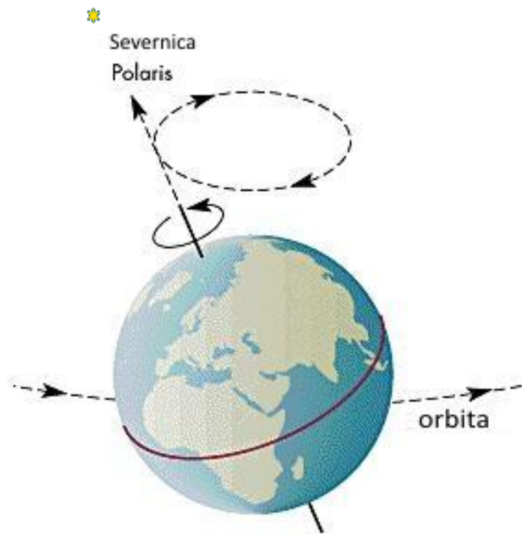
Zemljina rotacija osi danas
